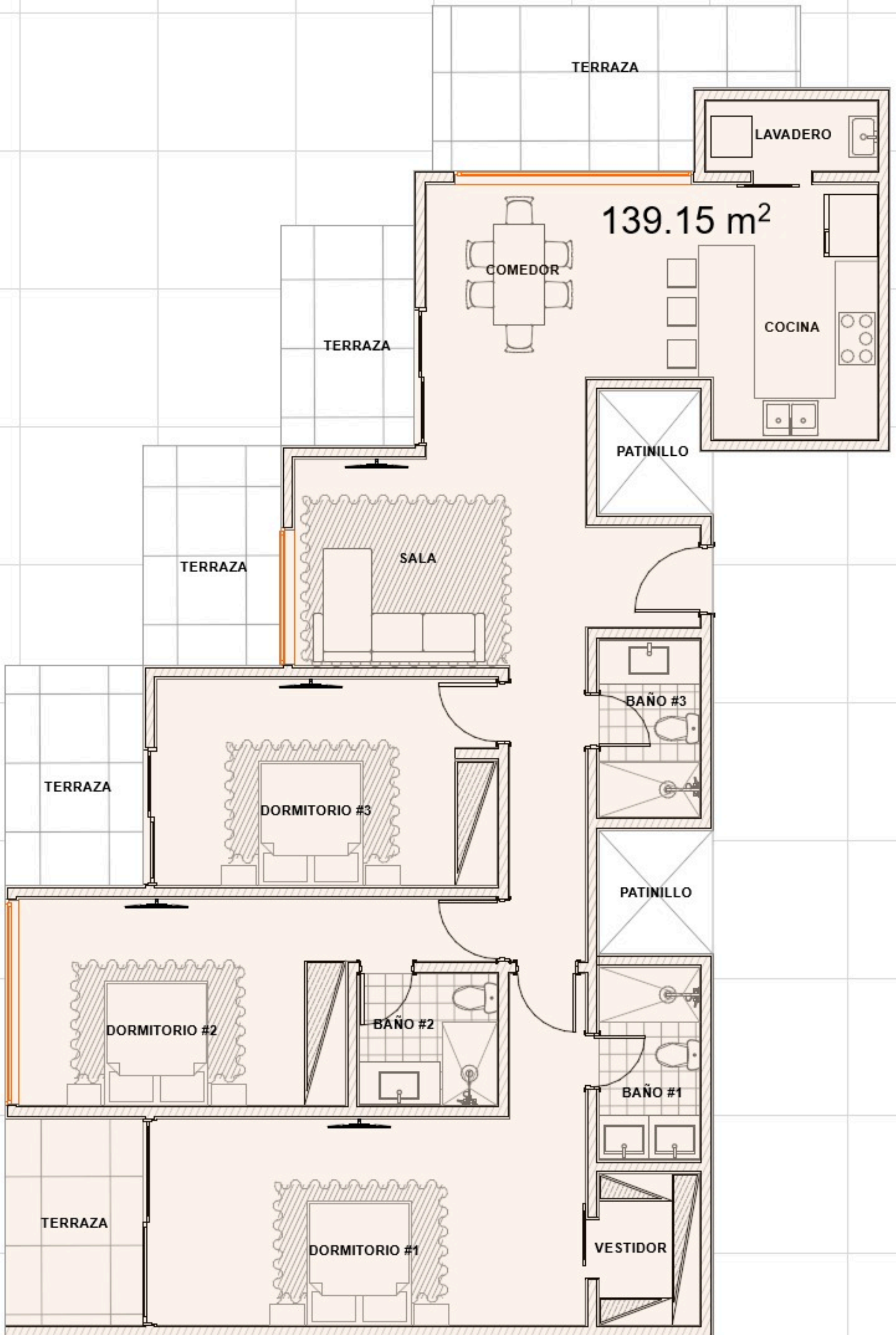
PLANO TIPO APART. E 4TO NIVEL (3 DORMITORIOS)
