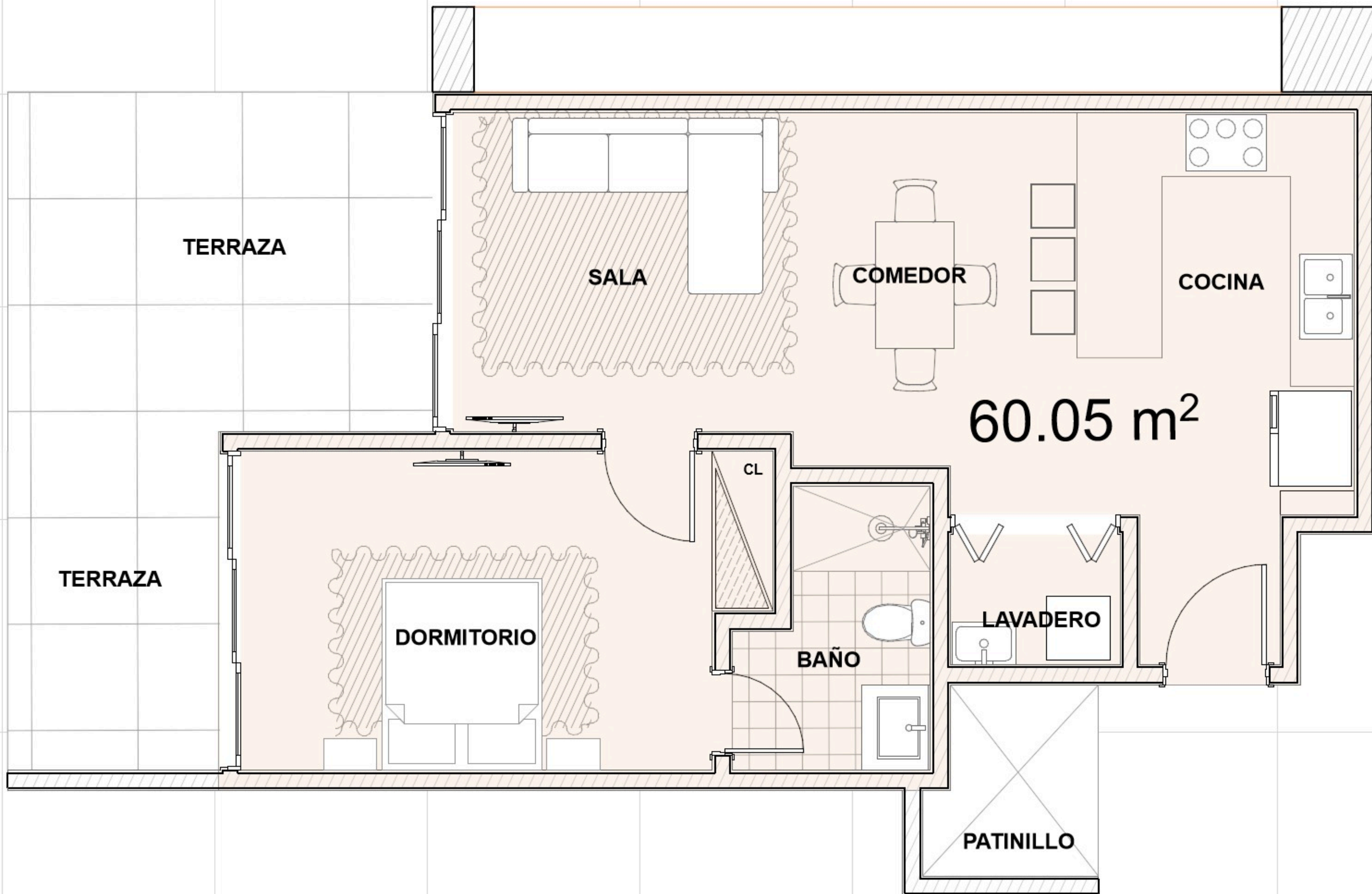
PLANO TIPO APART. C 2DO NIVEL (1 DORMITORIO)
