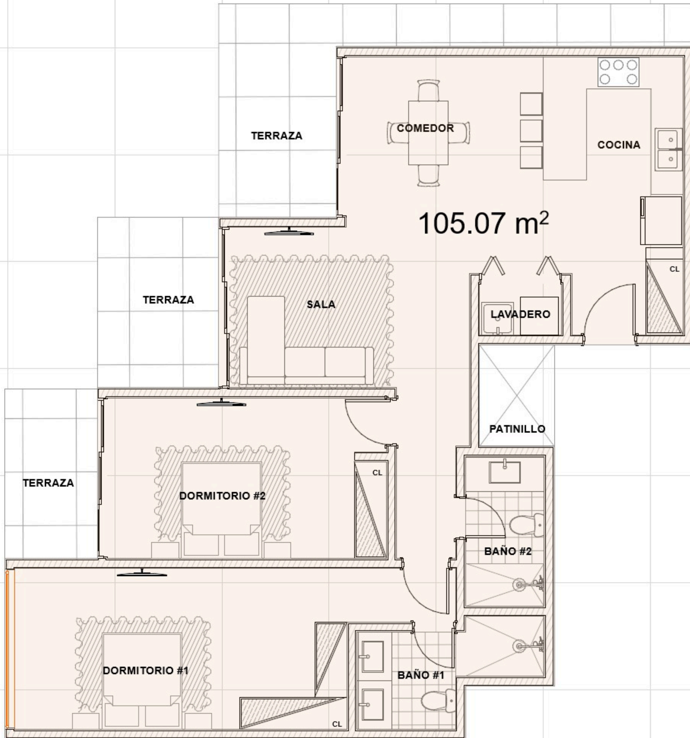
PLANO TIPO APART. D 3ER NIVEL (2 DORMITORIOS)
